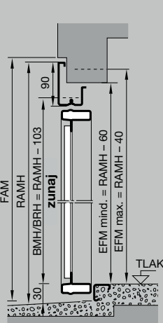
Montaža z vložki za vrata s spodnjo pripiro
