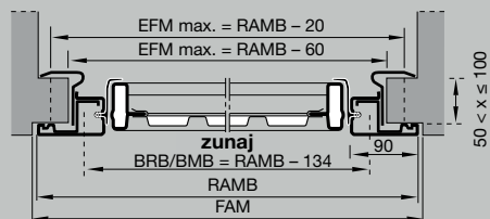
Montaža s sponkami (min. 50 mm, maks. 100 mm globine špalete)
