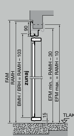
Montaža s sponkami brez spodnje pripire
