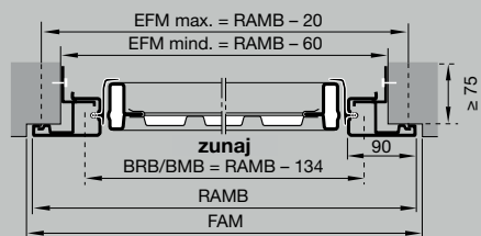
Montaža s sponkami (min. 50 mm, maks. 100 mm globine špalete)
