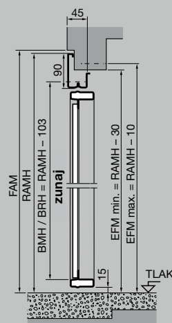
Montaža z vložki brez spodnje pripire
